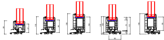
Porte fenêtre avec seuil bas
